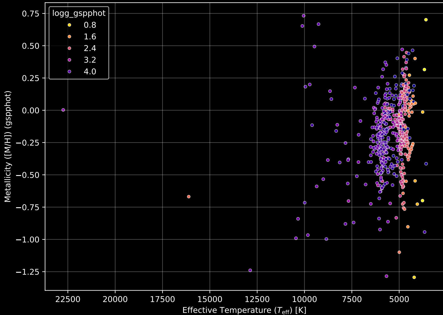
APOGEE DR17 Field: [K05_080+14] Stellar Population Parameters (n= 573)
